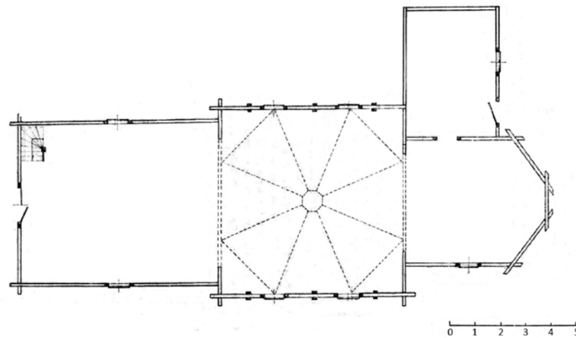
Ryc. 51. Rzut cerkwi w Dyniskach, wg J. Górkę 1984.
